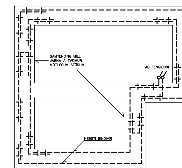
GRUNNMYND SÖKKULVEGGJA
