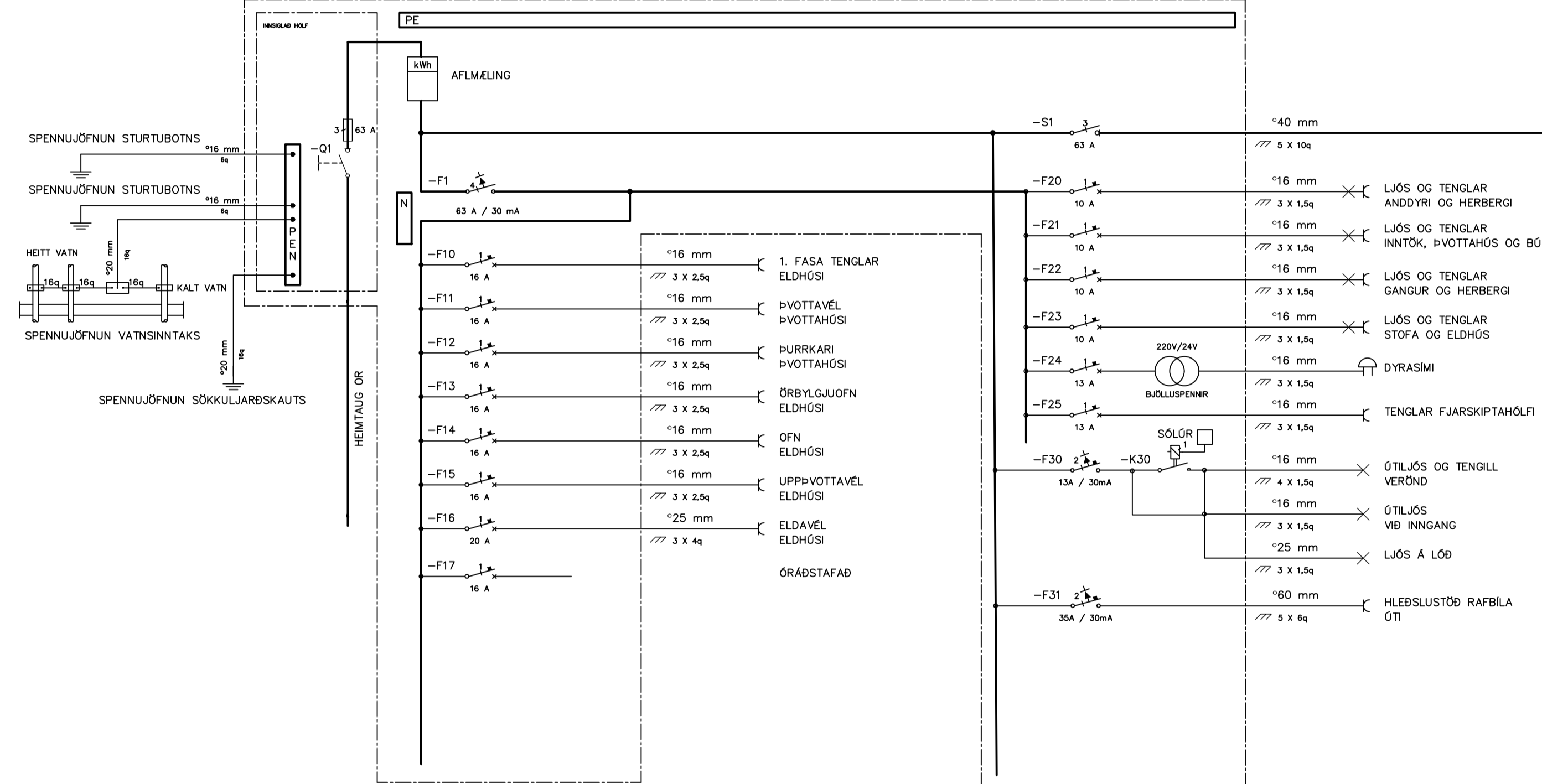
EINLÍNEMYND MÆLASKÁPAR +T2.1, +T4.1 OG T6.1
