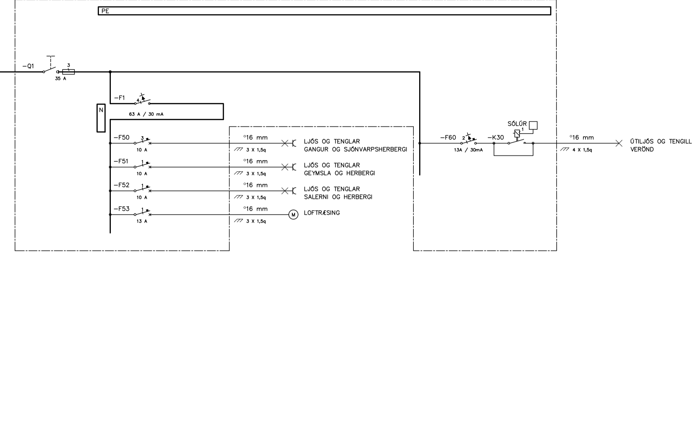
EINLÍNEMYND SKÁPAR +T2.2, +T4.2 OG T6.2
